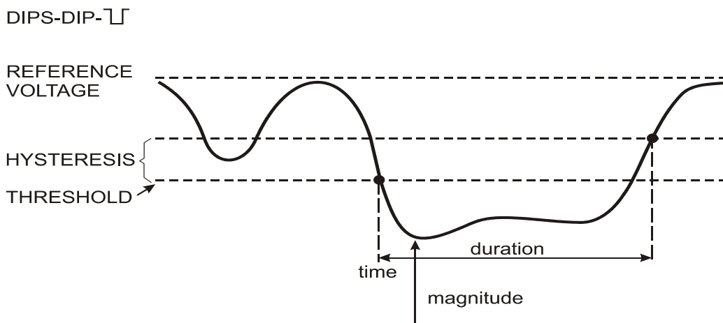
Obrázek 9-1. Charakteristiky poklesu napětí
