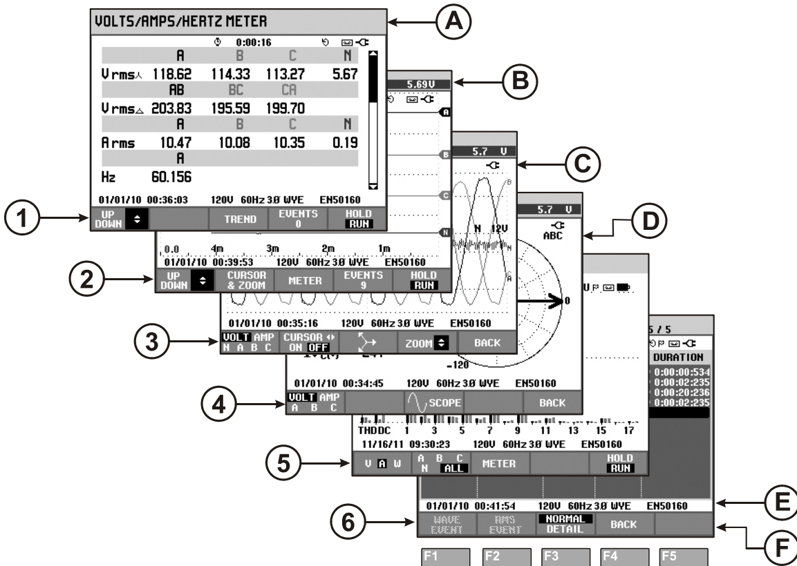
Obrázek 5-1. Přehled typů displeje
