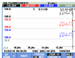
Obrázek 22-6. Obrazovka Trend se zapnutým kurzorem a zoomem
